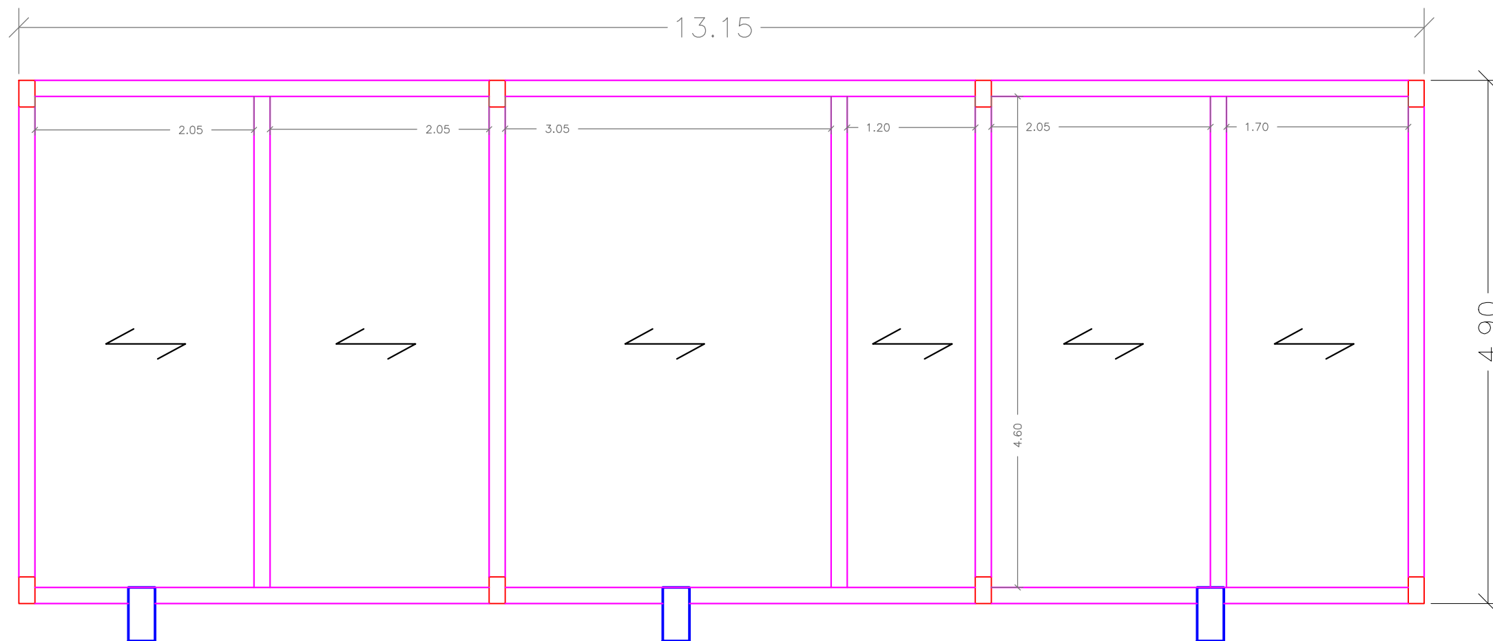
FORMAS LAJE DE COBERTURA – VESTIÁRIOS E SANITÁRIOS ÁREA=64,44m 2
