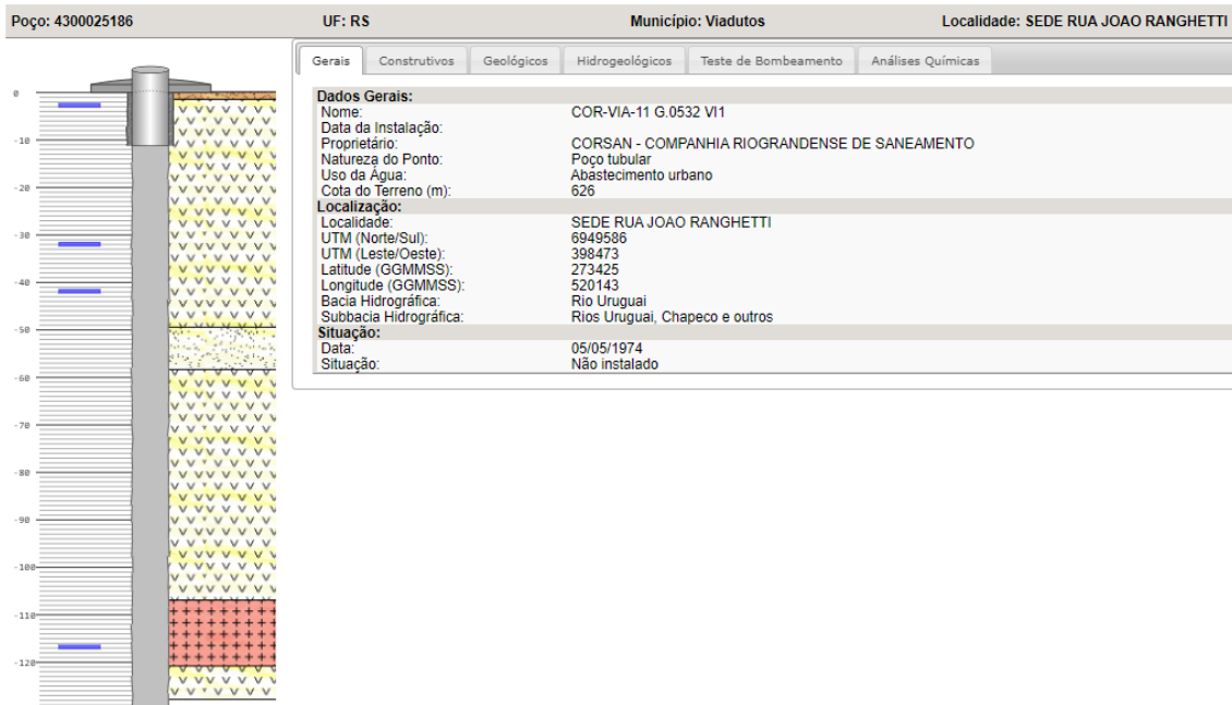
Figura 11: Perfil Geológico do Poço 2. Fonte: SIAGAS (2024).
