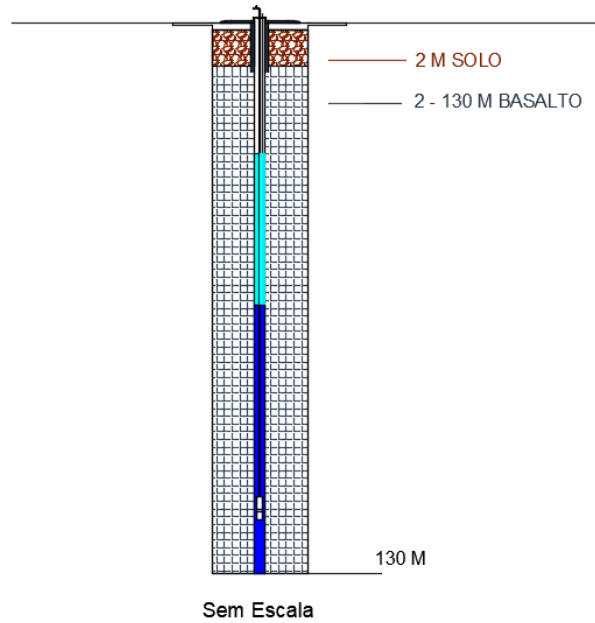
Figura 12: Perfil Geológico do Poço. Fonte: Autor (2024).
