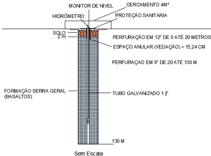
Figura 13: Perfil Construtivo do Poço. Fonte: Autor (2024).
