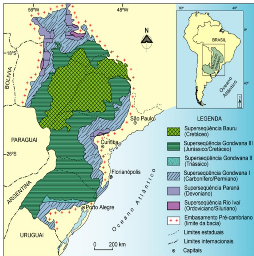
Figura 1: Mapa da Área da Bacia do Paraná. Fonte: Modificado de Milani (1997).
