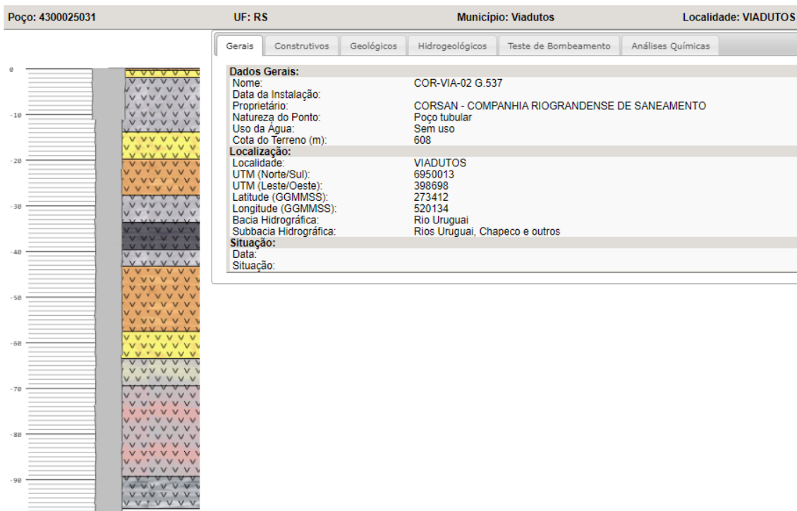
Figura 10: Perfil Geológico do Poço 1. Fonte: SIAGAS (2024).
