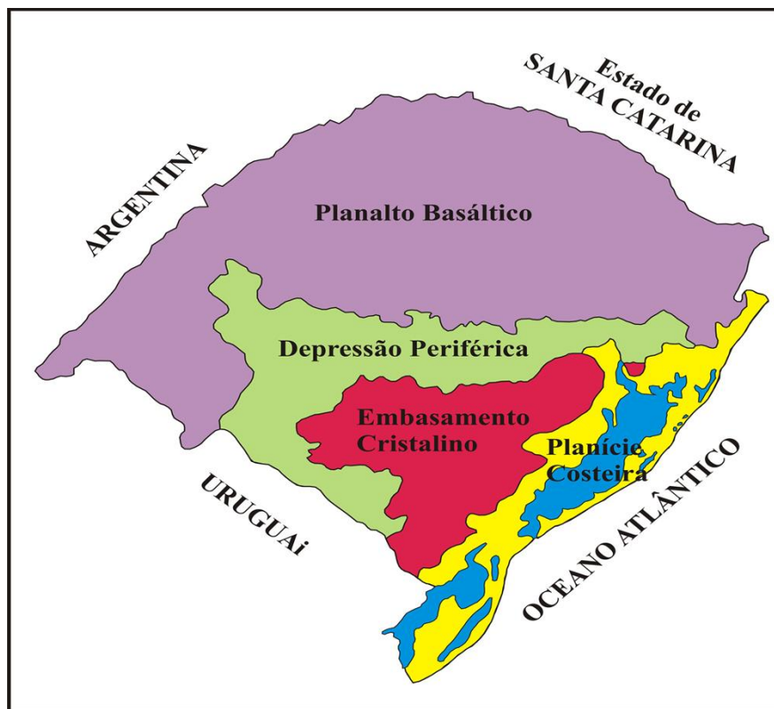
Figura 3: Províncias Geomorfológicas e Geológicas do Rio Grande do Sul.
