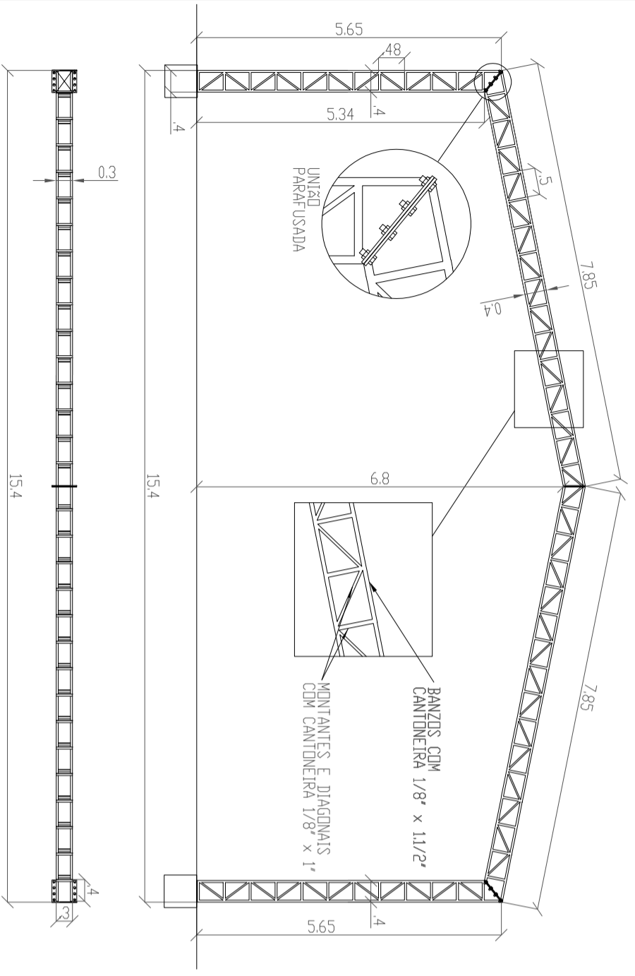
PÓRTICO SIMPLES - AV. BRASIL
