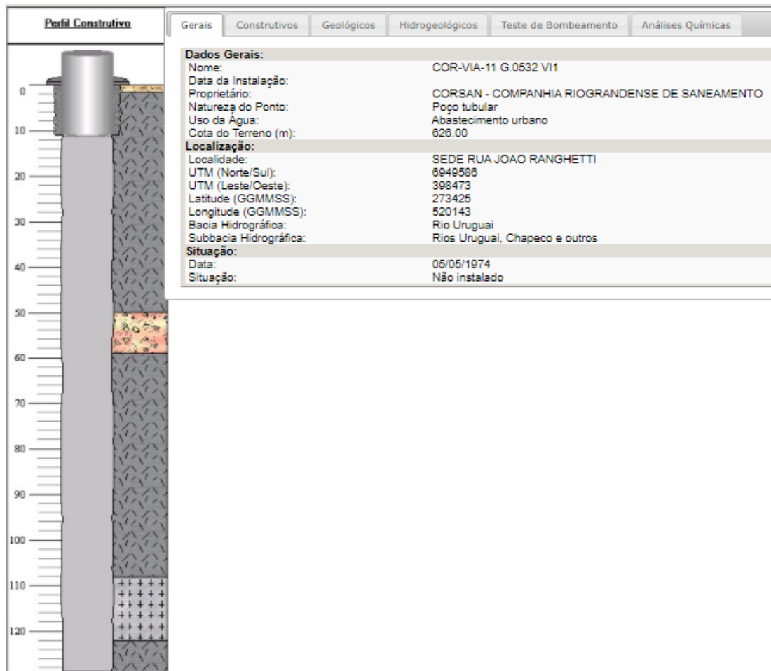
Figura 11: Perfil Geológico do Poço 2. Fonte: SIAGAS (2021).
