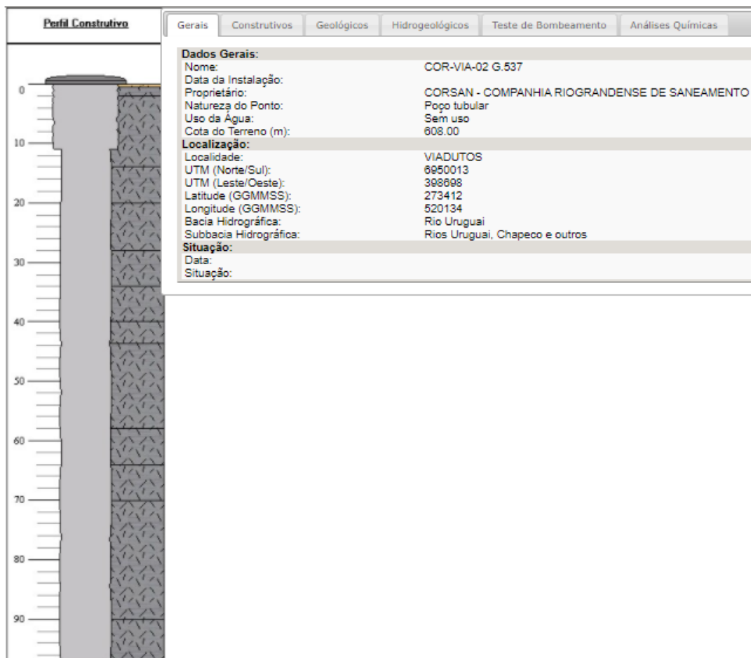
Figura 10: Perfil Geológico do Poço 1. Fonte: SIAGAS (2021).
