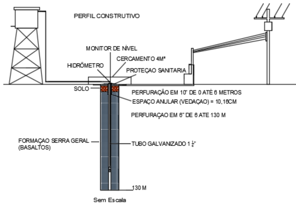
Figura 13: Perfil Construtivo do Poço. Fonte: Autor (2021).
