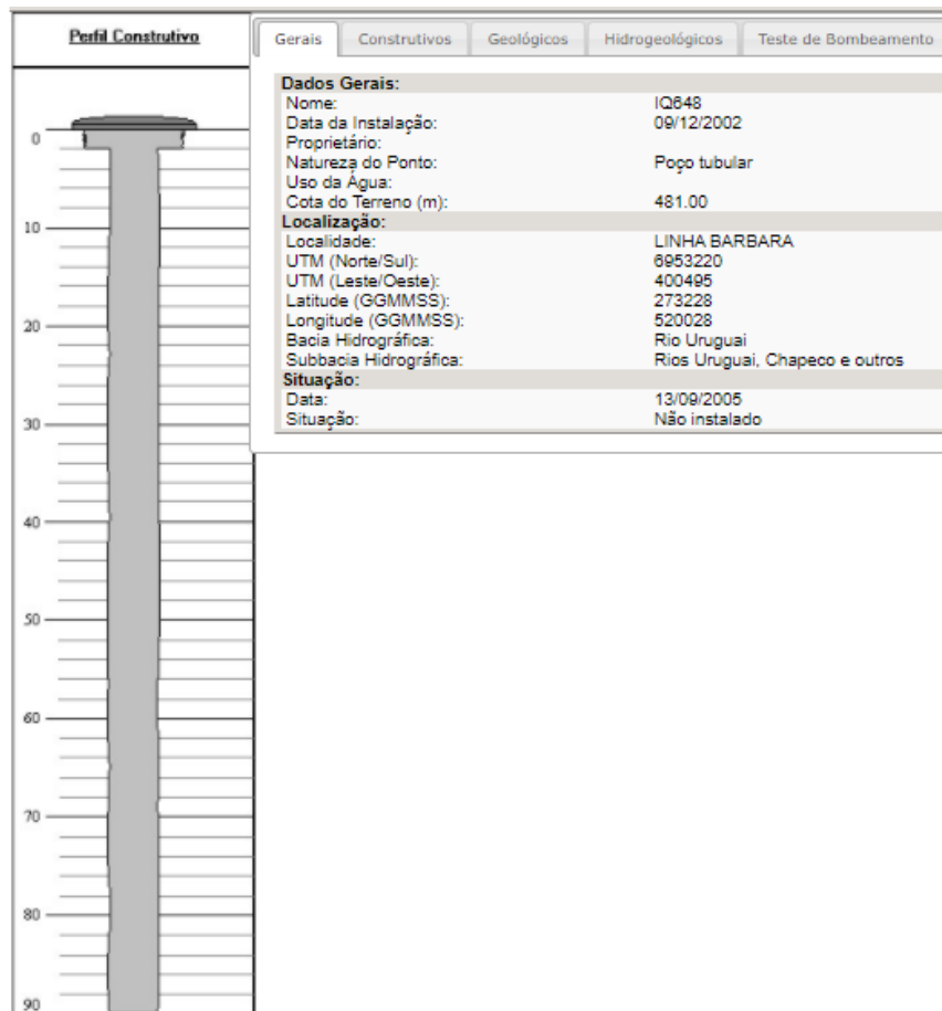
Figura 12: Perfil Geológico do Poço 3. Fonte: SIAGAS (2021).
