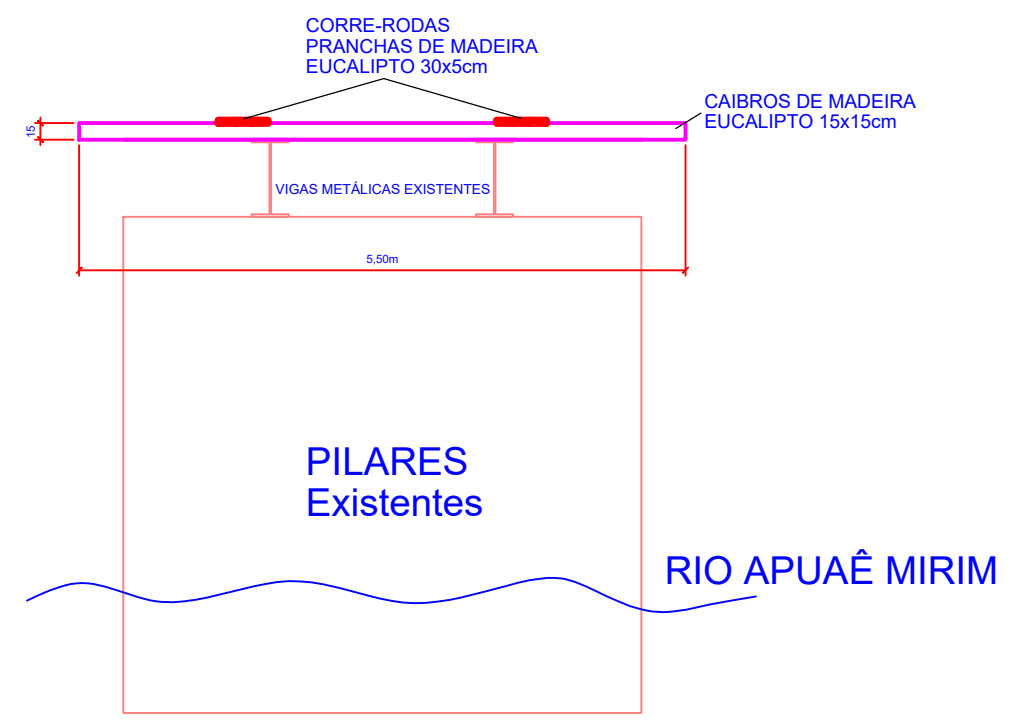
Corte BB
